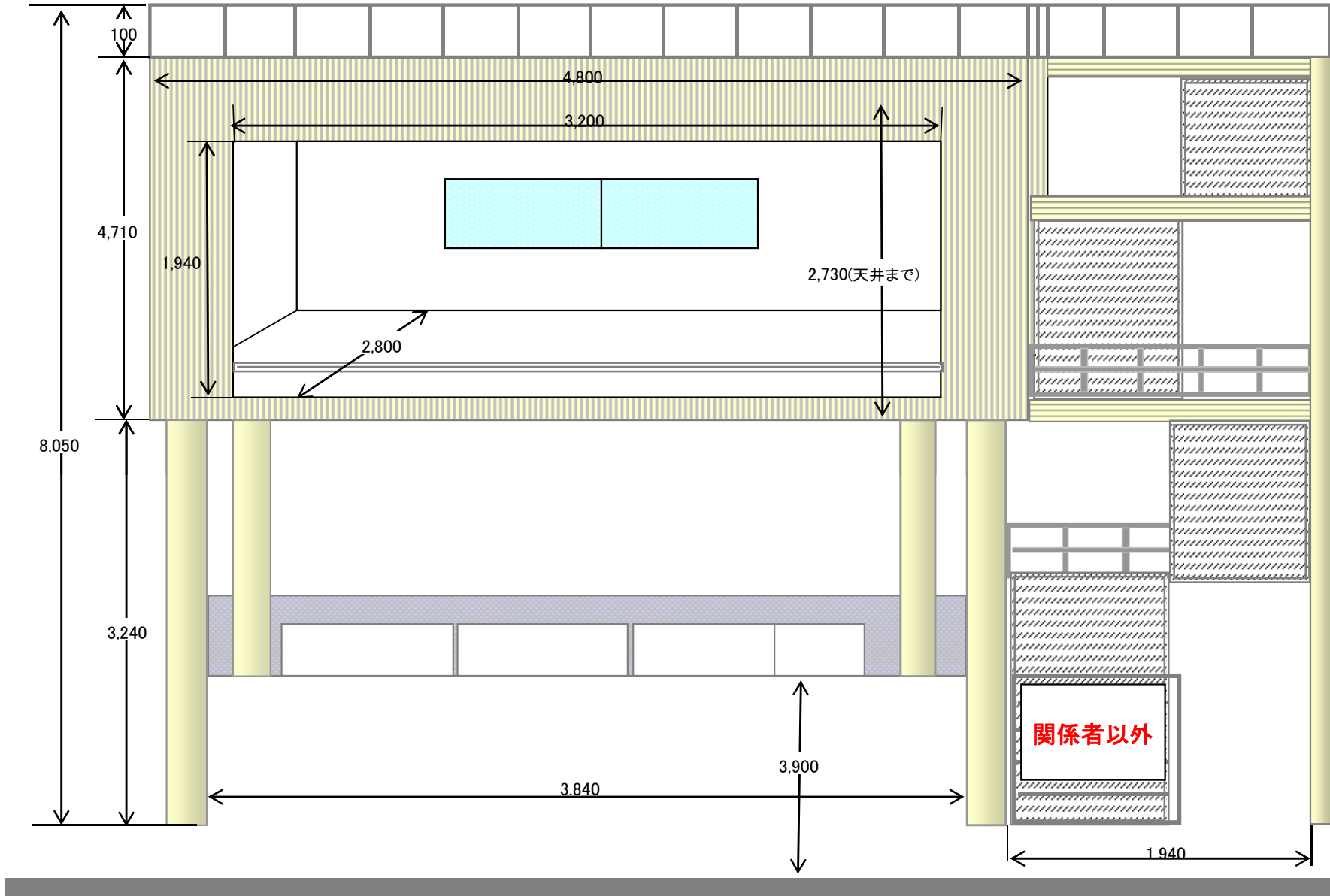
大阪城音楽堂(ピンタワー)断面図
